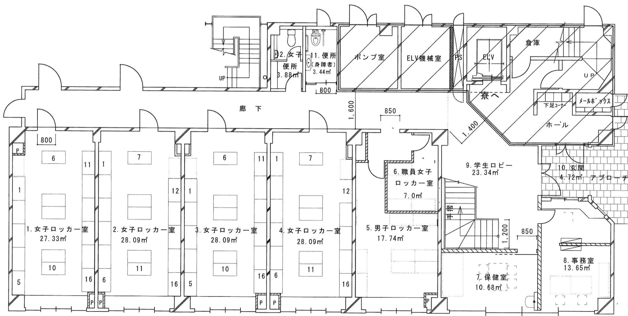
別館 1 階平面図
